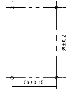
取付穴加工寸法 1/2
