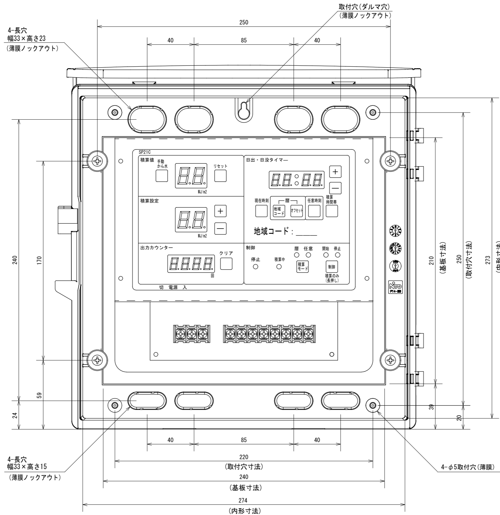
外形寸法 1 (1:2)
