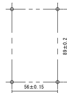
取付穴加工寸法 1/2
